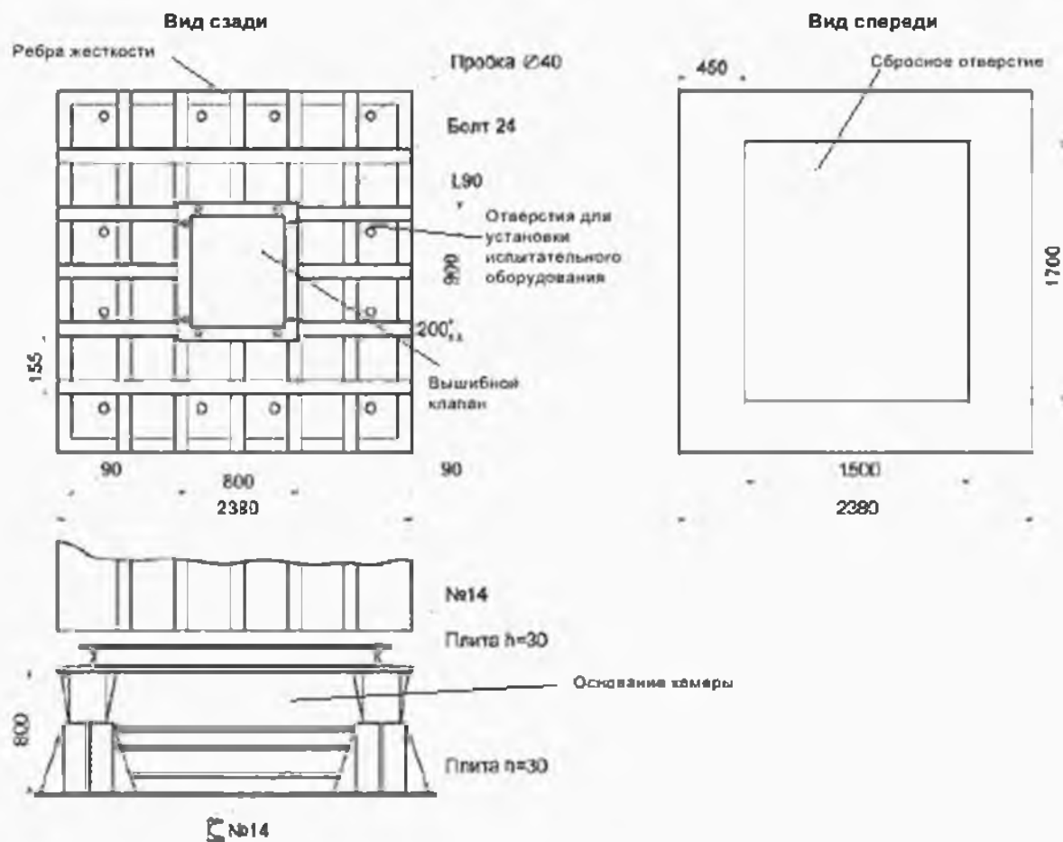
Рисунок А.1 – Схема испытательной взрывной камеры
